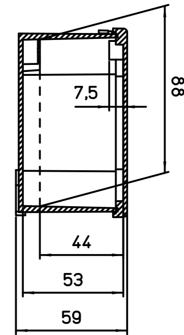
Sez. A-A
